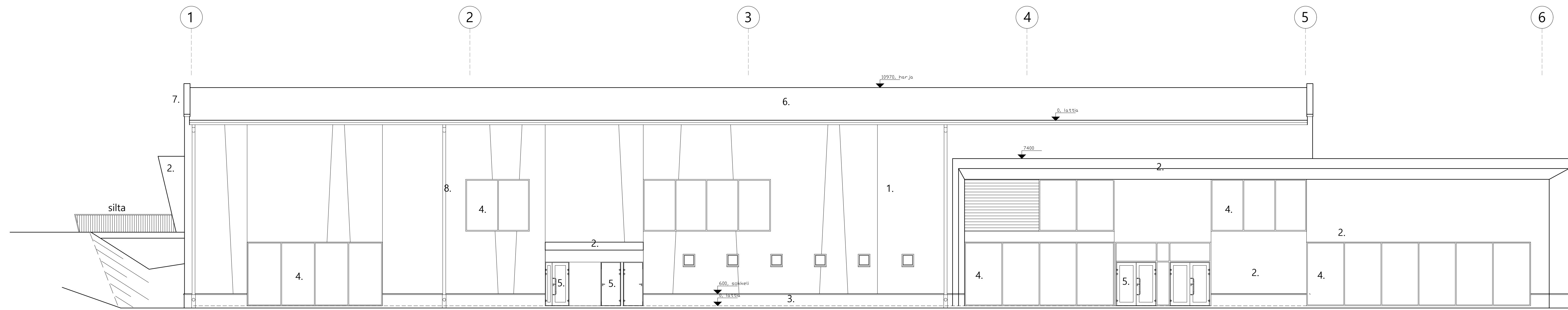
julkisivu luoteeseen
