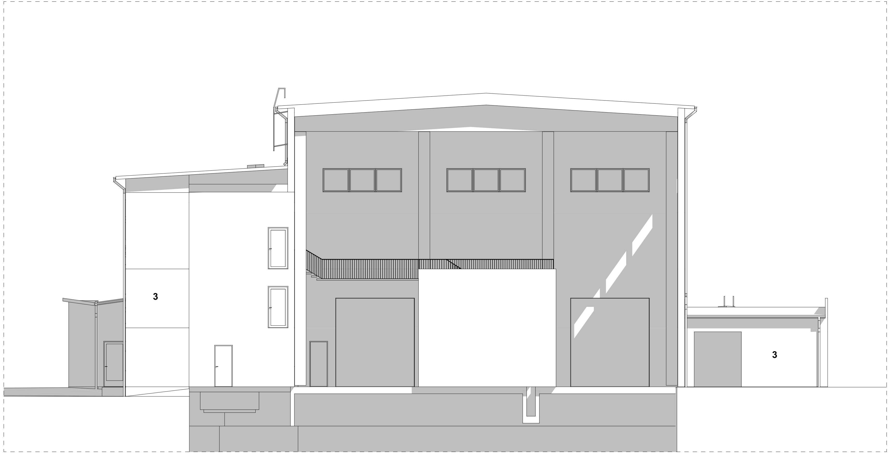
Julkisivu luoteeseen
