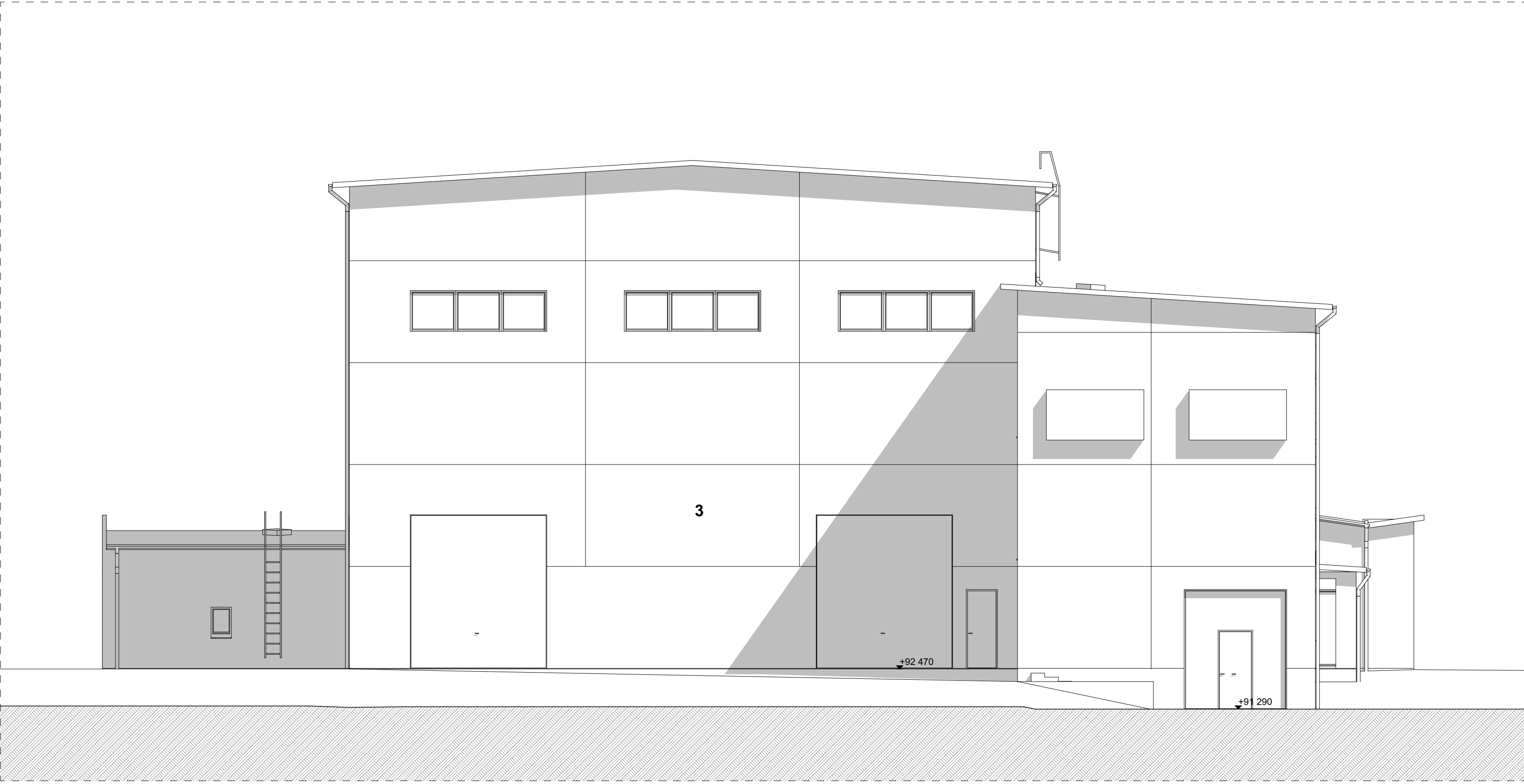
Julkisivu kaakkoon
