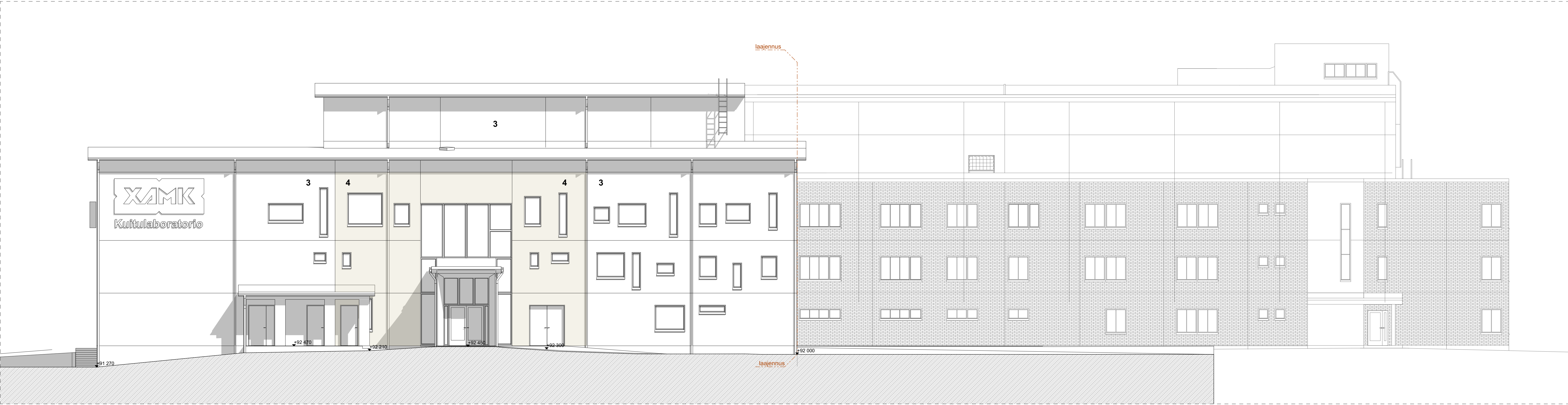
Julkisivu koilliseen
