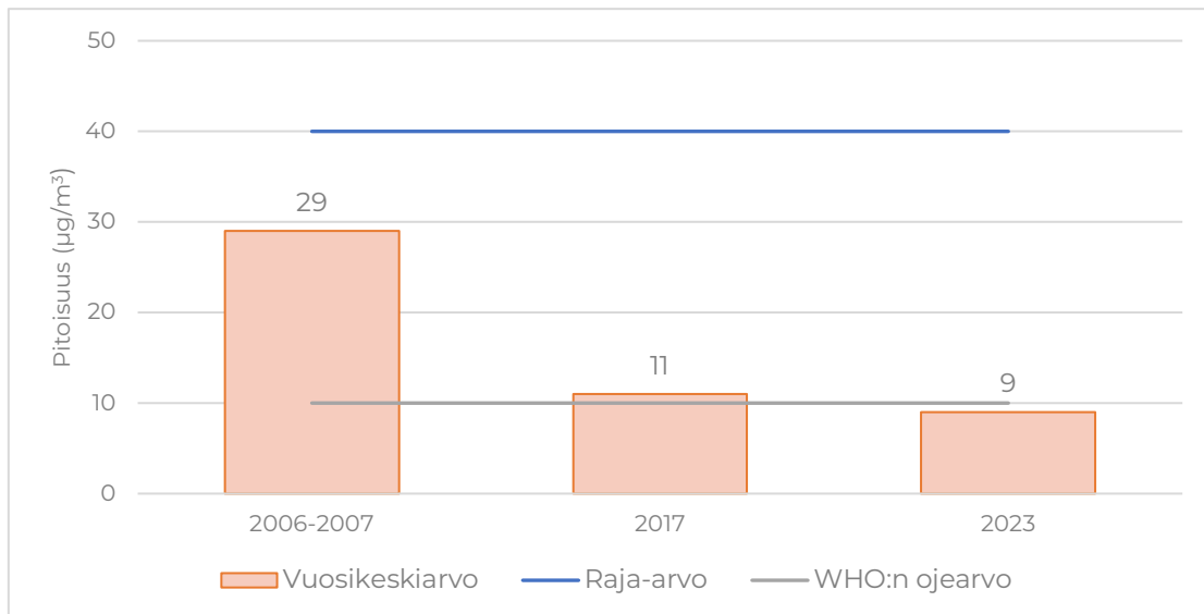
Kuva 21. Typpidioksidin vuosikeskiarvot suhteessa ilmanlaadun raja-arvoon ja WHO:n ohjeeseen Savonlinnassa vuosina 2006–2007, 2017 ja 2023.
