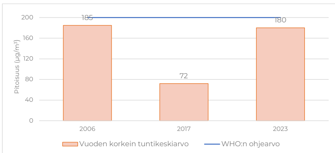
Kuva 18. Typpidioksidin tuntiarvo suhteessa WHO:n ohjearvoon Savonlinnassa vuosina 2006–2023.
