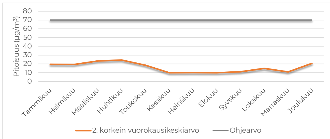
Kuva 16. Typpidioksidin vuorokausiarvot suhteessa kansalliseen vuorokausiohjeeseen Olavinkadulla vuonna 2023.
