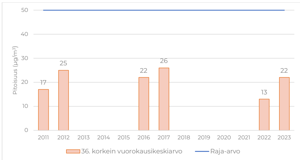
Kuva 12. Hengitettävien hiukkasten pitoisuudet suhteessa ilmanlaadun raja-arvoon Savonlinnassa vuosina 2011–2023.
