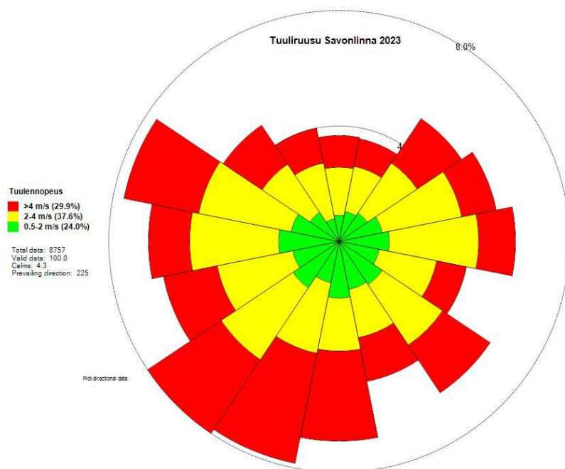
Kuva 7. Tuulen suunta ja nopeus Savonlinnassa vuonna 2023.
