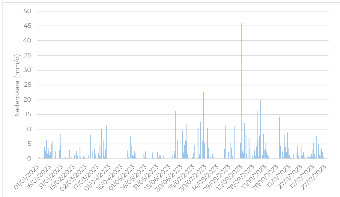
Kuva 5. Sademäärä Savonlinnassa vuonna 2023.
